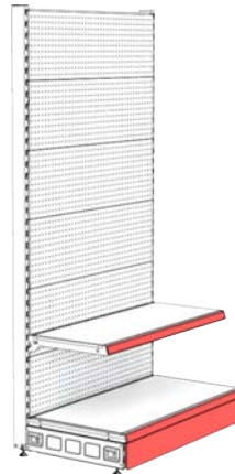
DUVAR ÜNİTESİ B500 4X300
