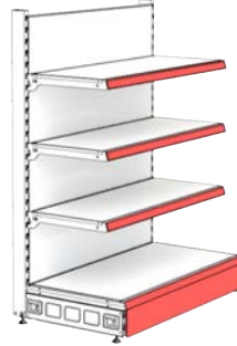
DUVAR ÜNİTESİ B500 3X400
