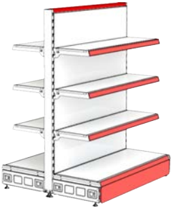
ORTA ÇİFTLİ ÜNİTE B400 3X300
