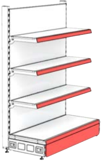
DUVAR ÜNİTESİ B400 3X300
